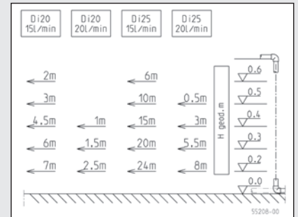
Schema hoogtes / afstanden
